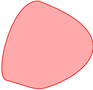
Рис. 1.10. Односвязная область
