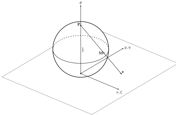
Рис. 1.1. Стереографическая проекция
