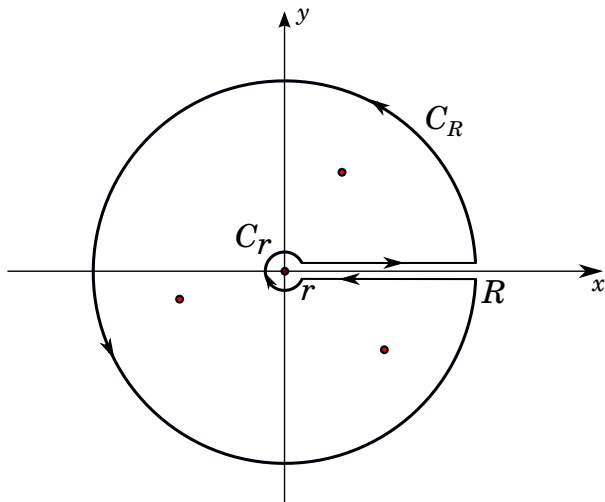
Рис. 5.1. Контур \Gamma_{r,R} .
