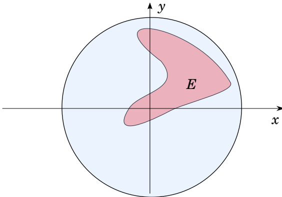
Рис. 1.12. Ограниченное множество.
